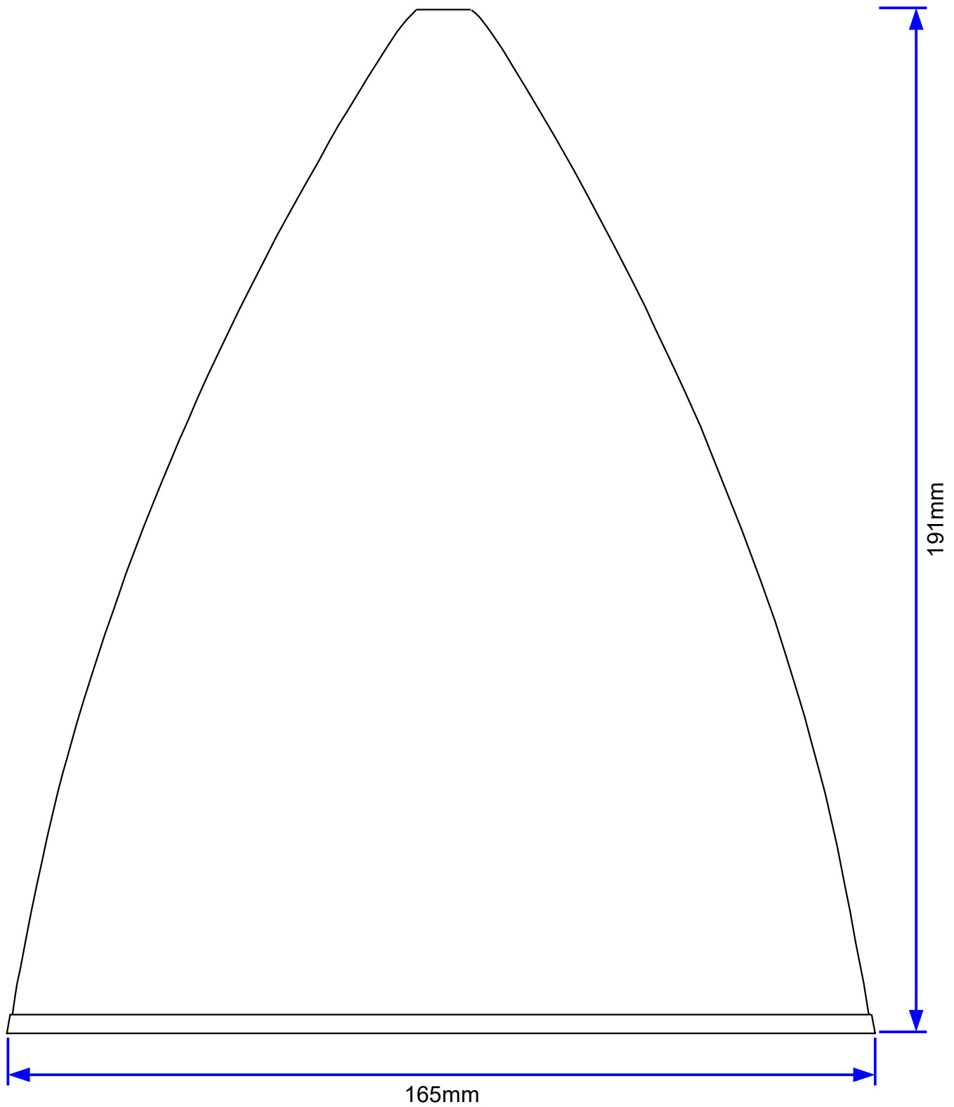
Spinner 165mm ø / 191mm Lang Best. Nr. 2165
